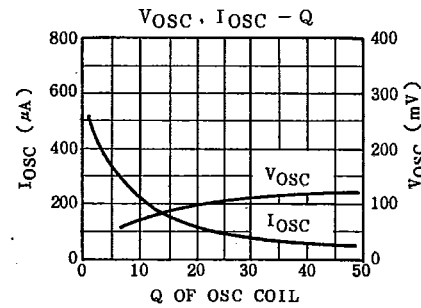
Graph 1 VOSC, IOSC - Q
