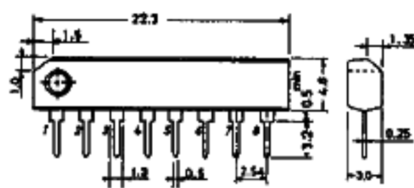
外形図 No.30168-581C (unit:mm)
